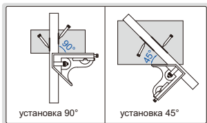
установка 90°
