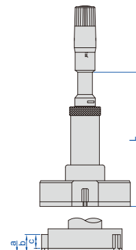
тип D 50-300 мм, твердосплавные точки измерения трехточечные
