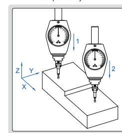
измерение глубины
