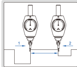
измерение длины
