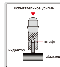
штифт ломается при достижении испытательного усилия 1580 кг
