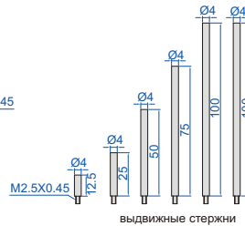
выдвижные стержни
