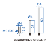
выдвижные стержни
