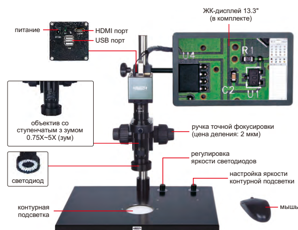
ISM-DL301 (с контурной подсветкой)
