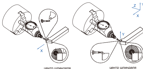
центр шпинделя
