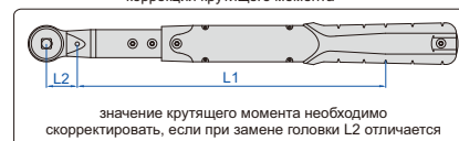
коррекция крутящего момента
