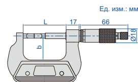
Тип В (мм)
