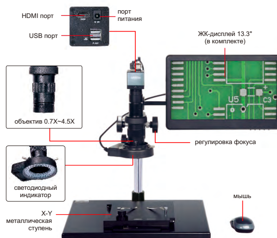
5318-MD60-XY (с подставкой)
