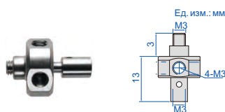
Многопозиционные основания M3 для щупов (мм)
