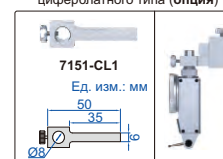
держатель тестового индикатора циферблатного типа (опция)
