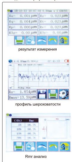
дисплей профилеометра
