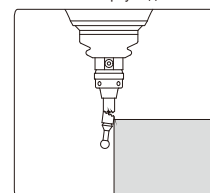
измерение глубины
