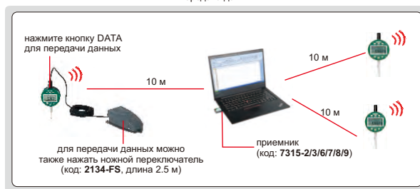
передача данных
