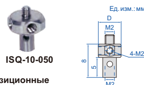
Многопозиционные основания M2 для щупов
