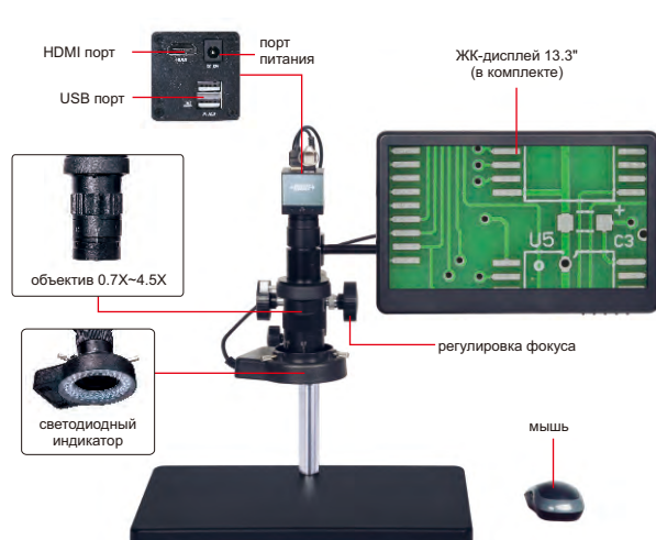
5318-MD60 (без подставки)
