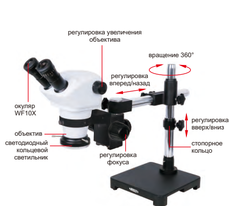
5106-M40 (с подставкой типа А)
