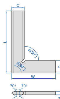
DIN875 класс 0 (мм)
