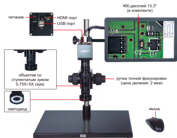
ISM-DL300 (без контурной подсветки)
